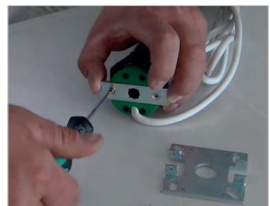
03 Motorkopfplatte anschrauben
